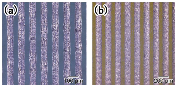
図 3. 開発した銅ナノペーストをフィルム上へスクリーン印刷した後、200 °C×30 min.焼成 (窒素雰囲気下の常圧焼成) して得られた配線状態図
