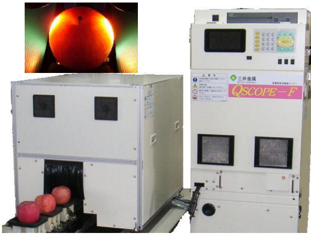
青果物非破壊内部品質センサ (Qscope-F)
